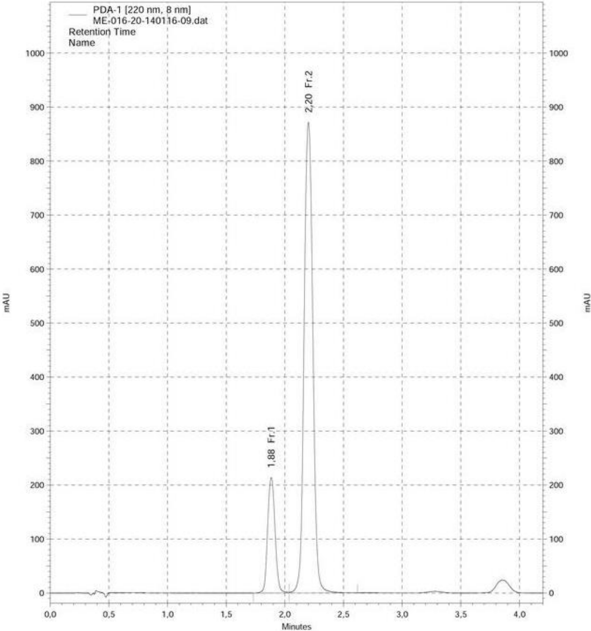
Analytische UHPLC-Trennung eines Substanzgemisches
